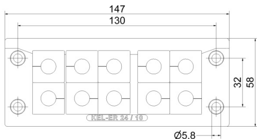
KEL-ER 24/10 , Art.No. SFKD-R001
