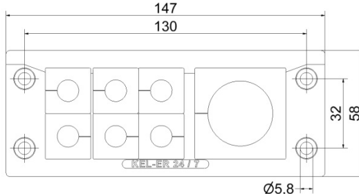
KEL-ER 24/7 , Art.No. SFKD-R002
